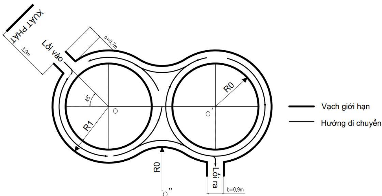
Hình 1: Hình bài sát hạch hình số 8
